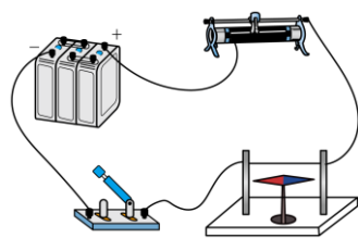
通电导线周围存在磁场
