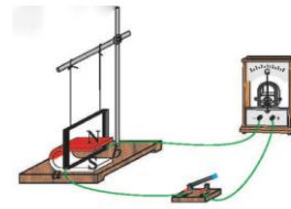
电磁感应现象
