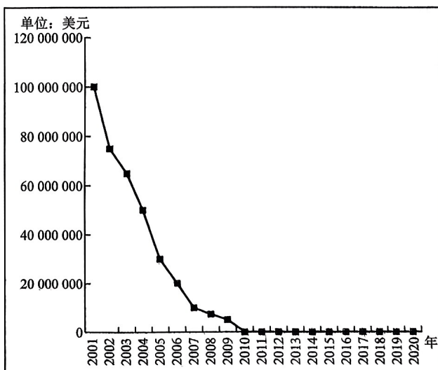
基因测序技术成本数据
