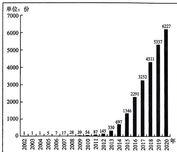
基因编辑技术研究论文发表情况
